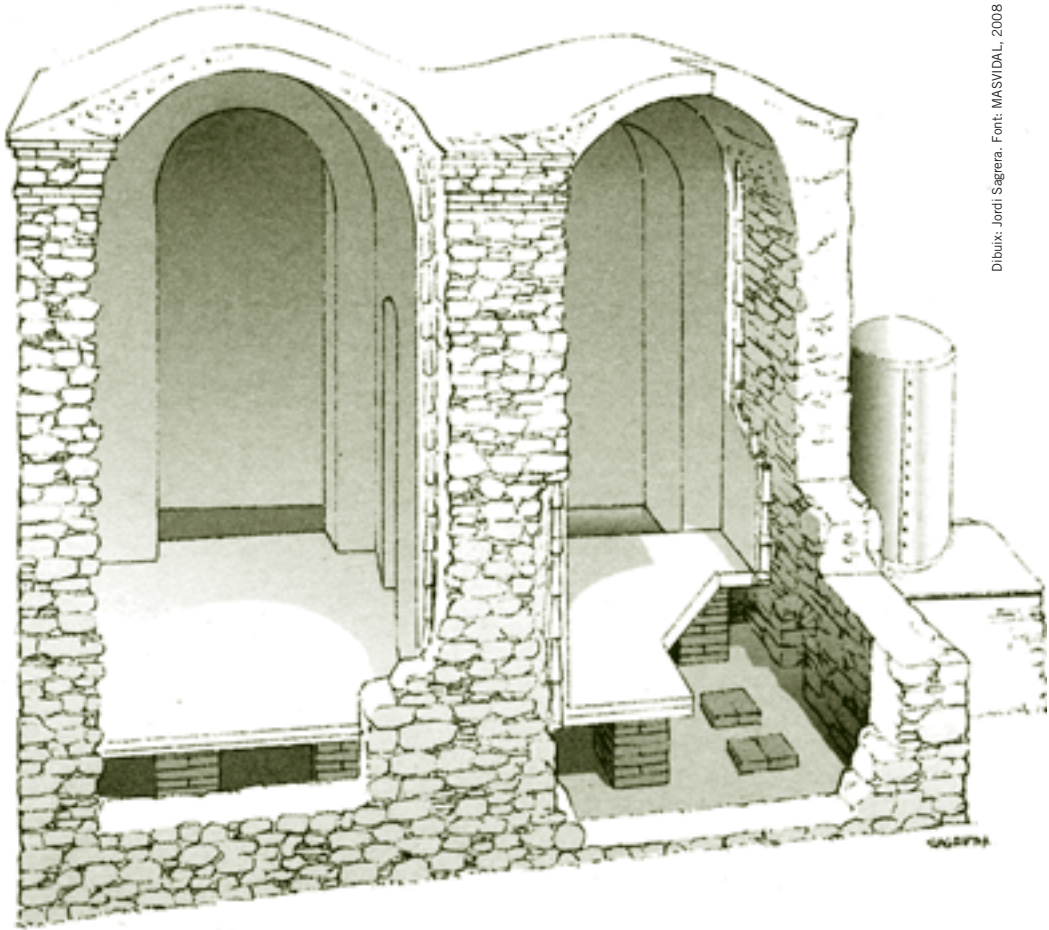
Figura 2.16. Restitució de l'edifici termal de la Torre dels Moros
