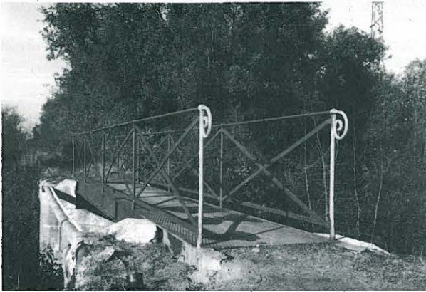
COL·LOCACIÓ DE LA PASSERA D'EN GOTARRA ON HI HAVIA EL «PONT DE FERRO».
