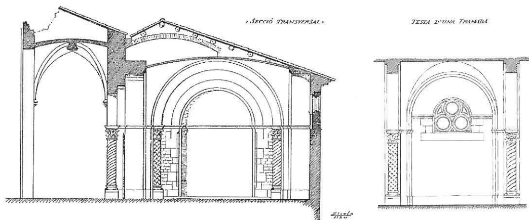
Secció transversal de la capella i les capelles laterals de l'Església on es pot apreciar el tipus de nau i l'alçada que Masó havia pensat per a la capella. (AHCAOC. Demarcació de Girona, Fons Rafael Masó).
